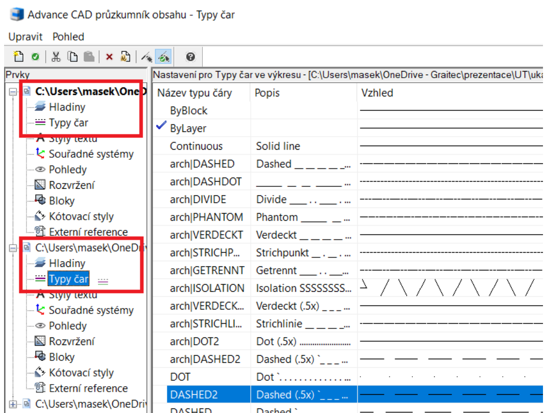
Ukázka přenosu typů čar z jednoho do druhého výkresu DWG.
